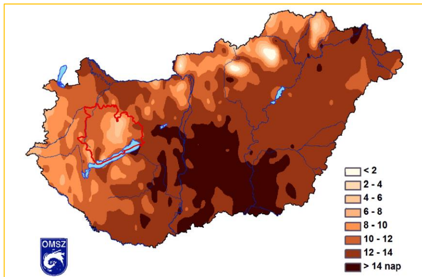
22. ábra: Hóhullámos napok száma (napi középhőmérséklet > 25^{\circ}\text{C} ) az 1981–2016-os időszakban
