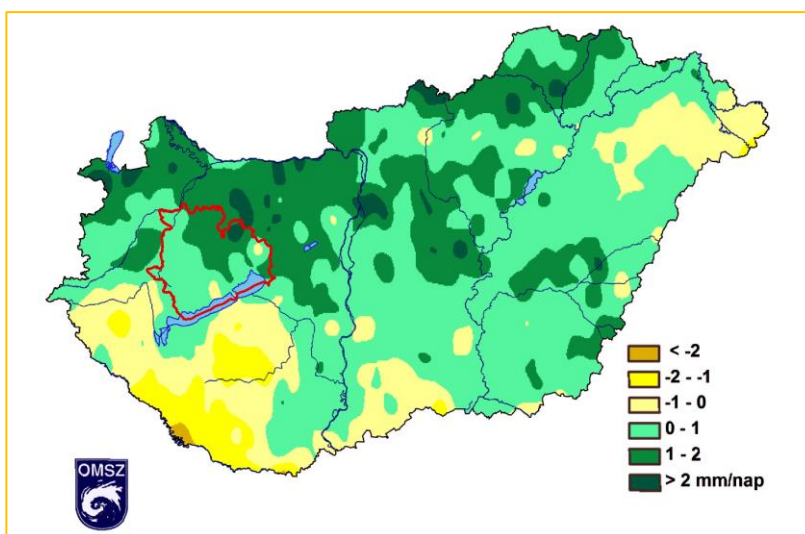
25. ábra: A nyári átlagos napi csapadékiintenzitás változása az 1961–2016 időszakban
