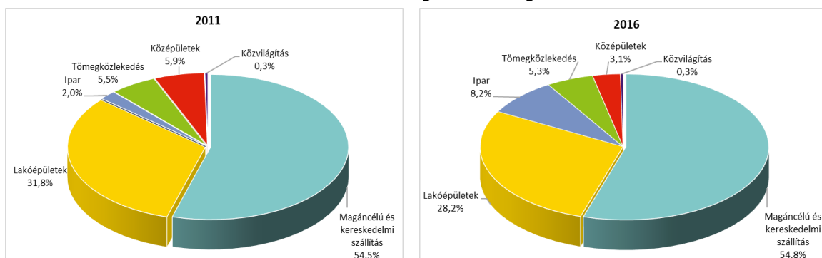
21. ábra: BAKONYÉRT Vidékfejlesztési Akciócsoport Egyesület Veszprém megyei működési területén keletkező üvegházhatású gáz kibocsátás
